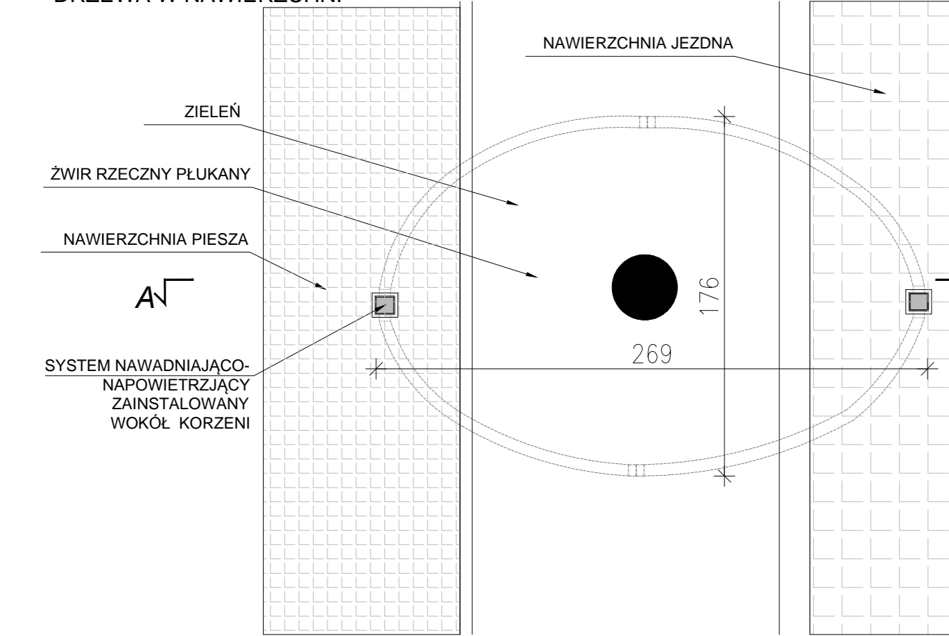
RZUT SCHEMAT
