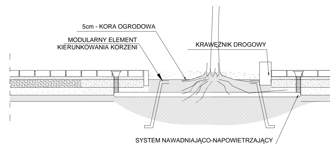
PRZEKRÓJ SCHEMAT
