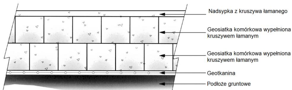
Rys. 10. Ściany oporowe wykonane z geosiatek komórkowych
