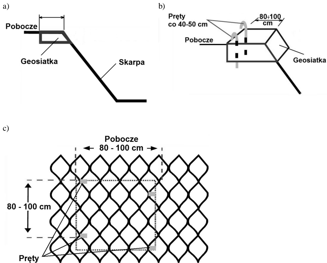
Rys. 12. Umocnienie skarpy geosiatką komórkową
