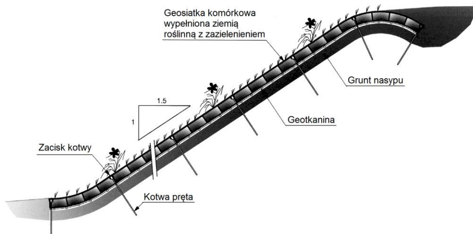
Rys. 13. Przykładowe przekroje poprzeczne utwardzonego pobocza, wykonanego przy użyciu geosiatki komórkowej
